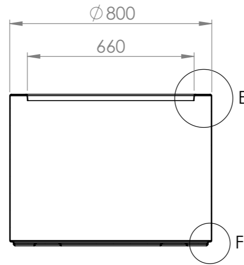
SECTION D-D SCALE 1 : 15
